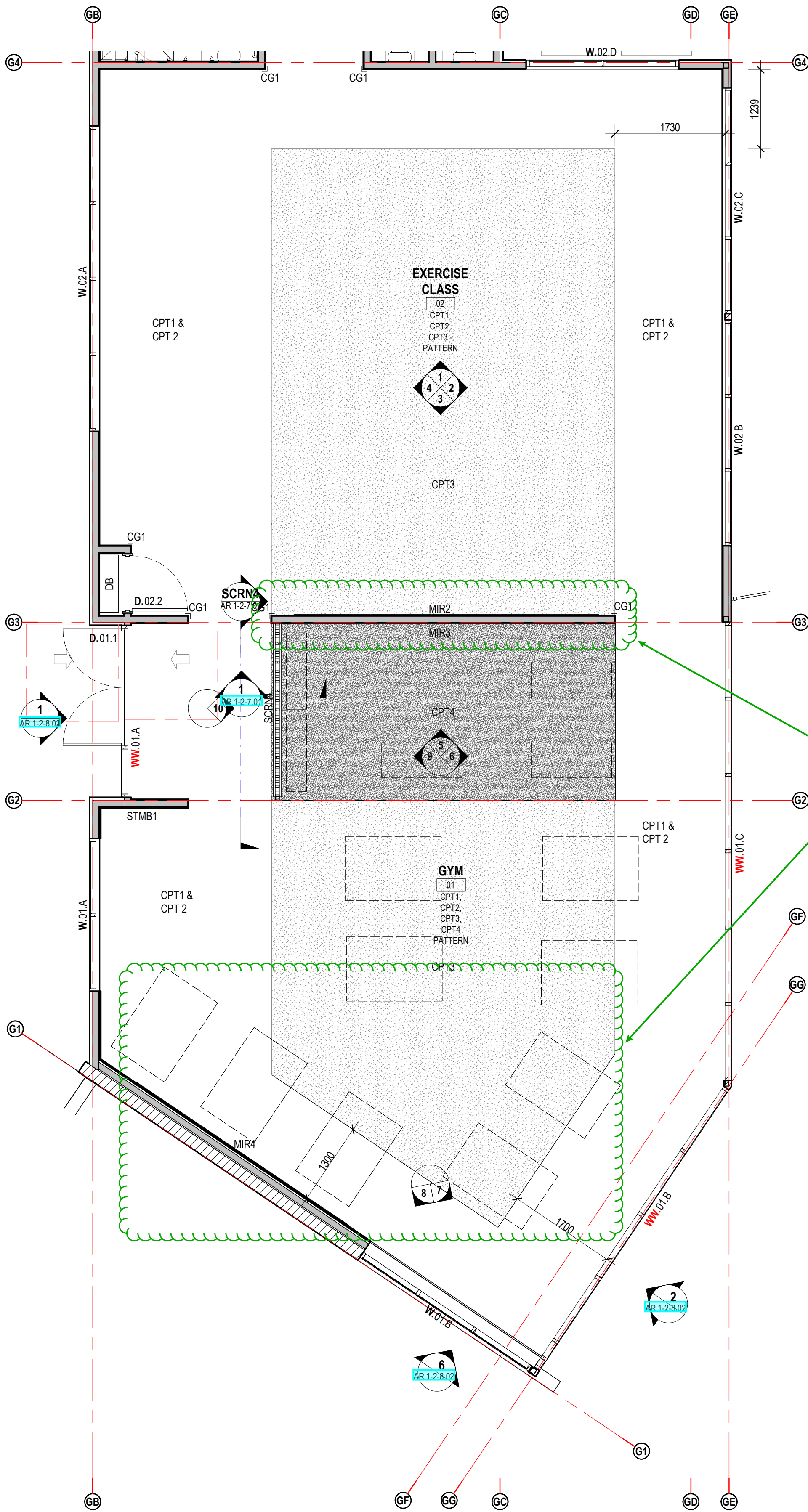
A GYM - FF&E PLAN 1 : 50
