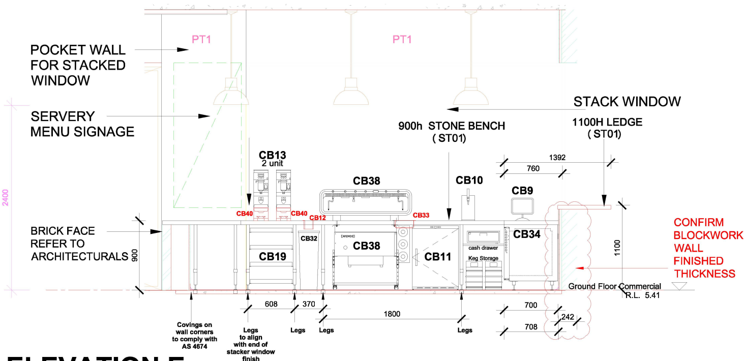
ELEVATION E
